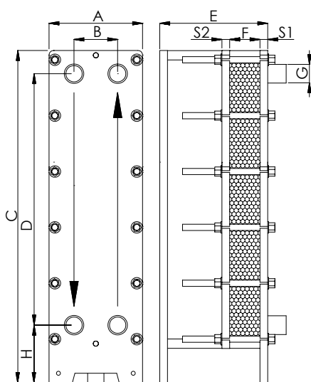
DIMENSIONEN
