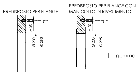
TIPO CONNESSIONI
