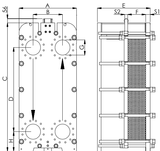
DIMENSIONI - INGOMBRI
