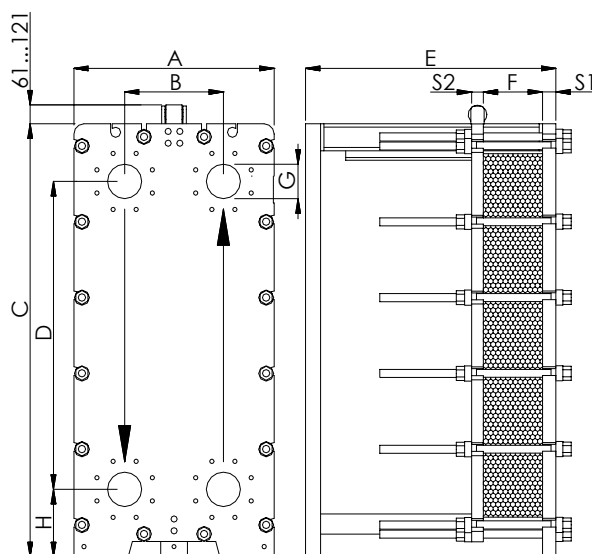
MEDIDAS TOTALES
