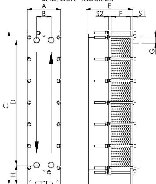
DIMENSIONI - INGOMBRI
