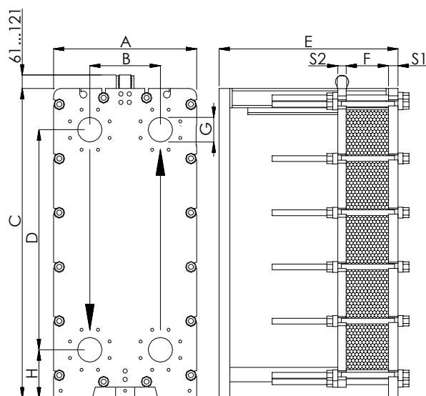
DIMENSIONI - INGOMBRI
