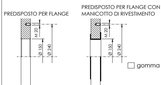
TIPO CONNESSIONI
